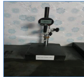
Đồng hồ đo độ sâu
