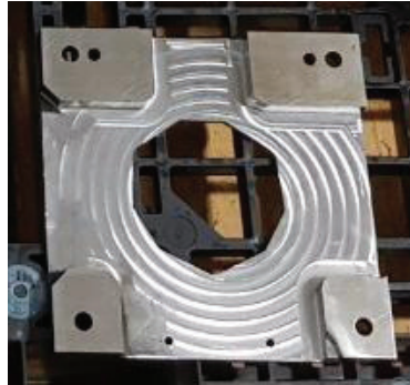
Chi tiết gá khuôn dập nguội
