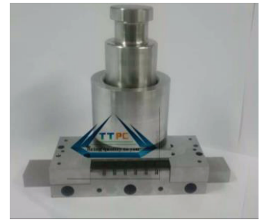
Cụm đồ gá ép cao su
