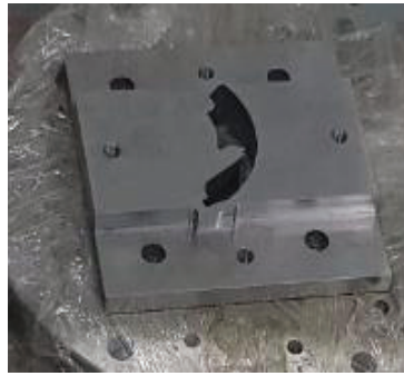
Chi tiết biên dạng cối dập nguội
