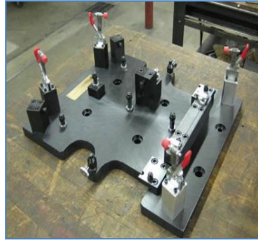
Cụm đồ gá 02
