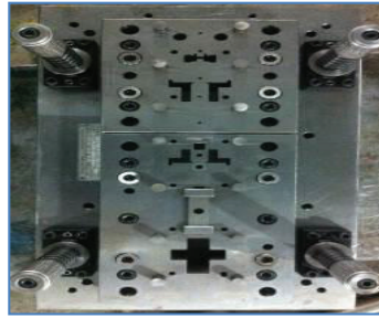
KDN liên hoàn 02
